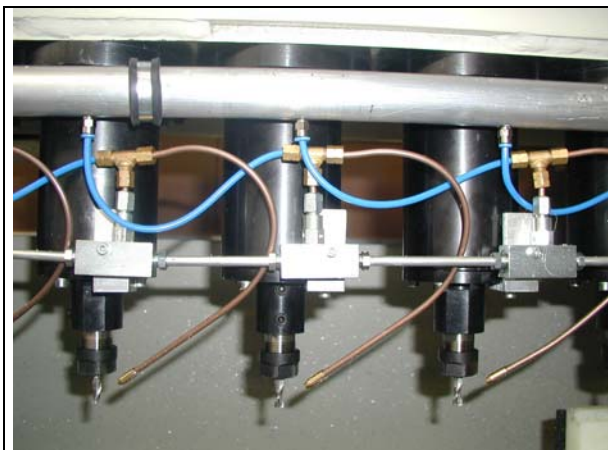
Spindels op vaste tussenafstand met olievereveling Broches à distance fixe avec lubrification par fumée d'huile Spindles at a fixed interval with oil mist lubrication Spindeln mit festem Zwischenabstand mit Ölvernebelung
