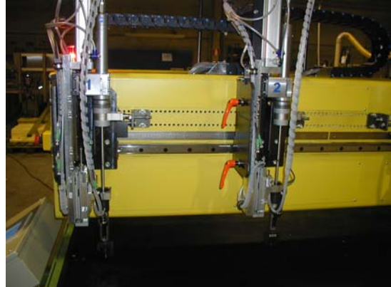
Positie van de schroevendraaiers is manueel verstelbaar La position des tournevis est réglable manuellement The position of the screw drivers is manually adjustable Die Position der Schraubenzieher ist manuell verstellbar
