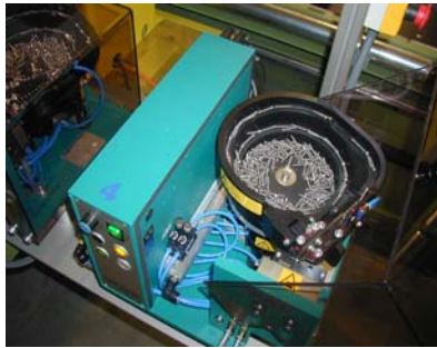
Trilkuip voor toevoer van de schroeven Bol vibrant pour alimentation de vis Bowl feeder for feeding the screws Wendelförderer führt die Schrauben an
